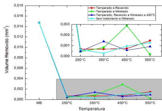
Figura 2- Volume de desgaste para amostras nitretadas a plasma
