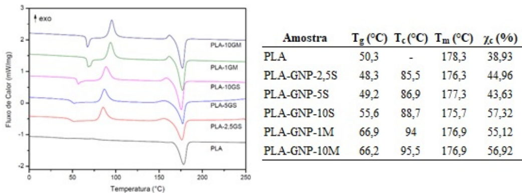
Figura 1 – Ensaio DSC PLA puro e Nanocompósitos
