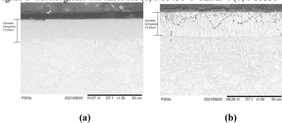
Figura 1- Metalografia das amostras (a) NIT450°C-TEMP e (b) NIT550°C-TEMP
