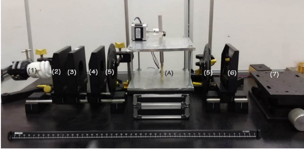
Figura 1: Fotografia do dispositivo para compressão de amostras fotoelásticas configurado no polariscópio linear por transmissão. (1) fonte de luz branca; (2) filtros e lentes; (3) filtro de cor; (4) polarizador linear horizontal; (A) amostra fotoelástica; (5) lâminas de 1/4 de onda; (6) polarizador linear vertical; (7) base para câmera digital.
