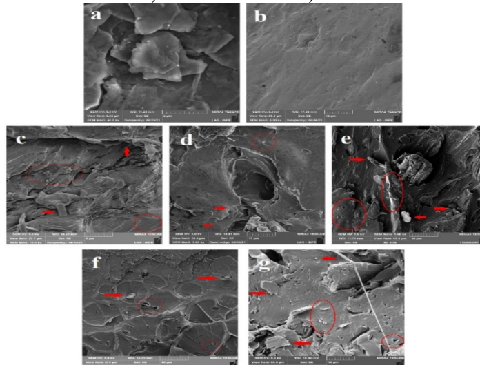
Figura 4 – Análise morfológica via FEG-MEV. a) GNP b) PLA c) PLA-GNP-2,5S d) PLA-GNP-5S e) PLA-GNP-10S f) PLA-GNP-10M
